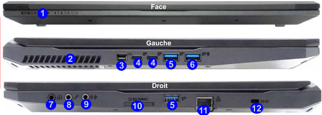
Figure 12 - Vues de face, gauche et droite (Modèle B)
