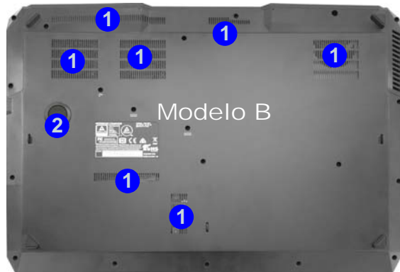
Figura 13 Vistas inferior y posterior (Modelos A & B)
